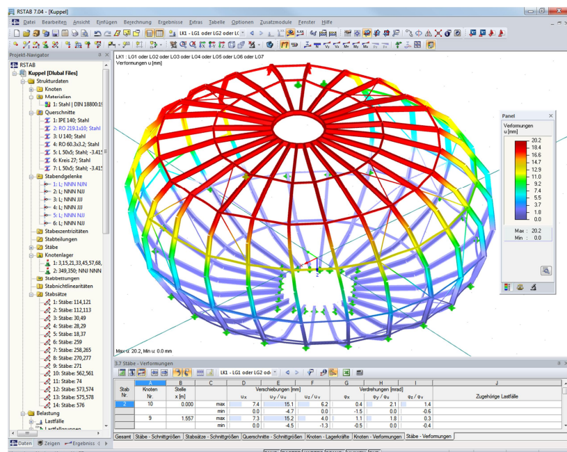
Verformungsbild der Dachkugelkonstruktion in RSTAB
