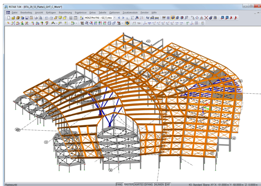
Teil der in RSTAB bemessenen Struktur (Screenshot: Dlubal)
